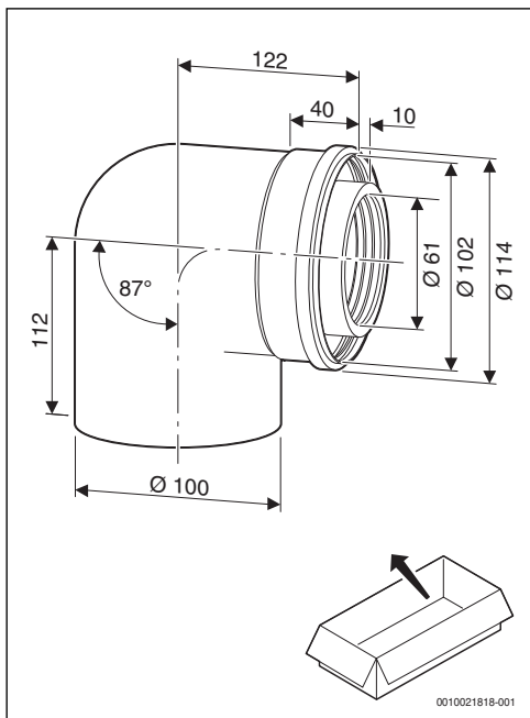
1 FC-CE60-87(-S)
