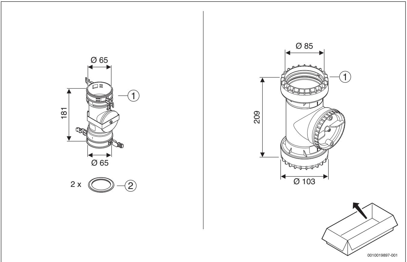
1 Ø 60 mm: 7738112633, Ø 80 mm: 7738112692
