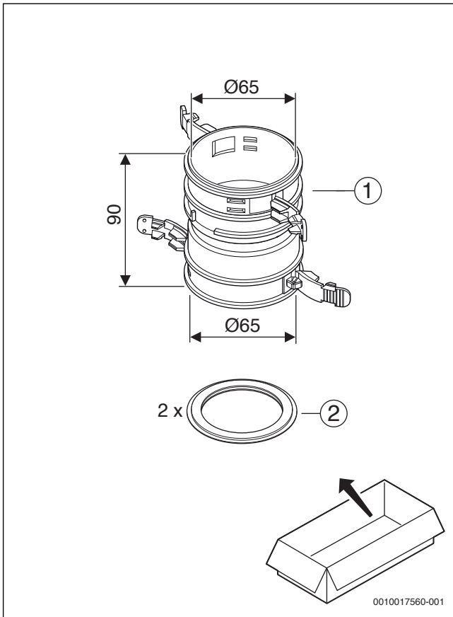
1 Ø 60 mm: 7738112634
